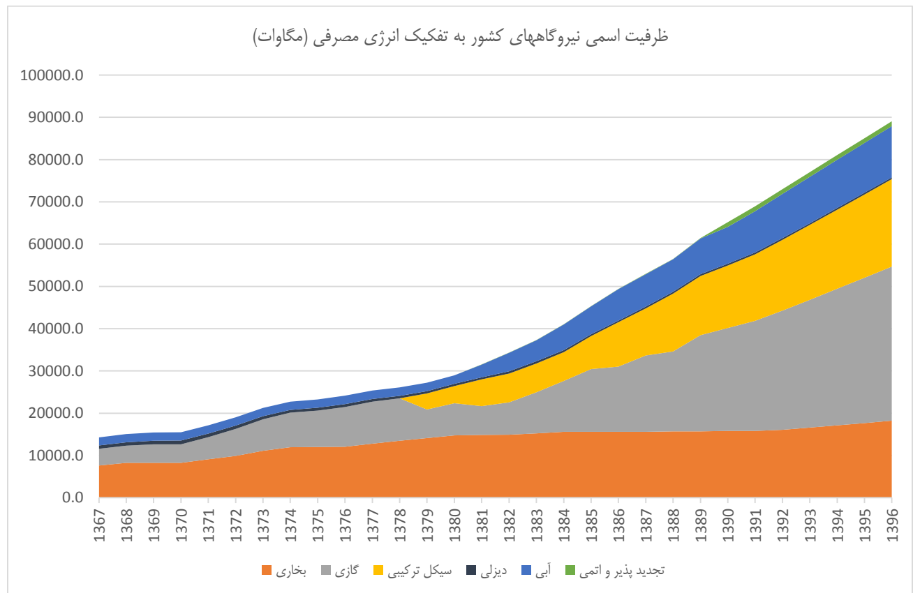
نمودار (۱) برون‌یابی روند ظرفیت اسمی نیروگاههای کشور به تفکیک انرژی مصرفی تا سال ۱۳۹۶
