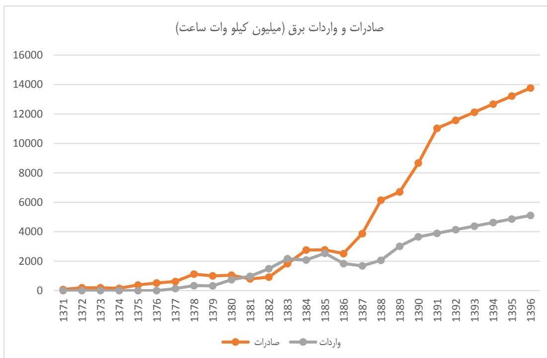
نمودار (۱۵) برونیابی روند صادرات و واردات برق تا سال ۱۳۹۶
